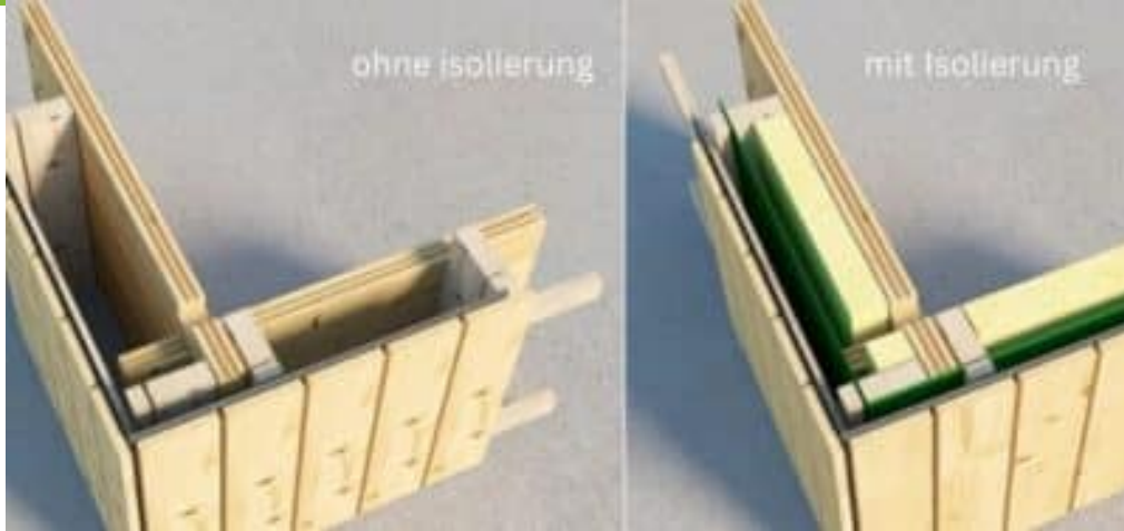
Holzverschalung
