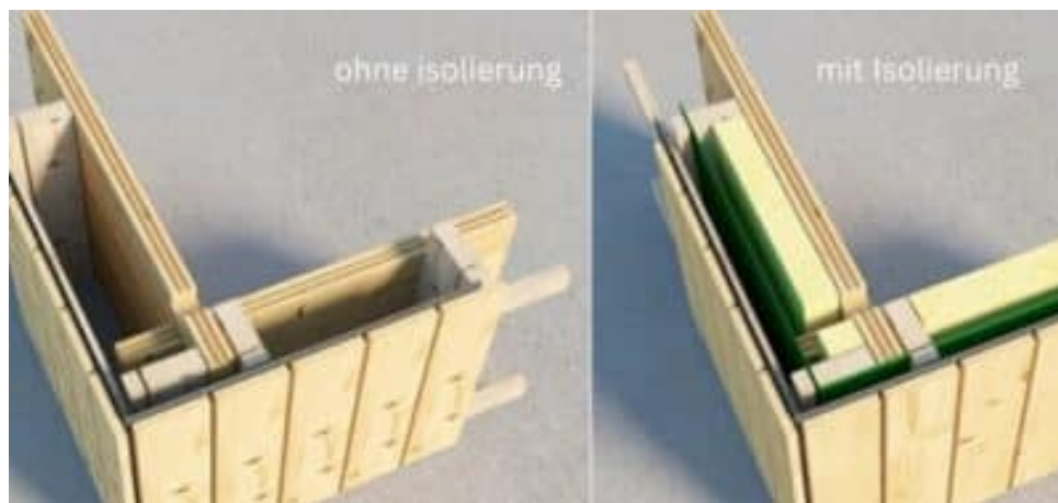
Holzverschalung
