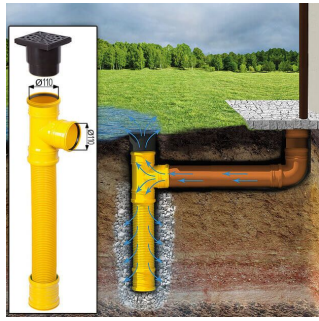
Sickerschicht mit Zufluss/Abfluss Ø 110 mm
